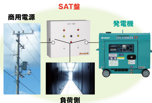
簡易自動始動盤 (SAT盤)※2
