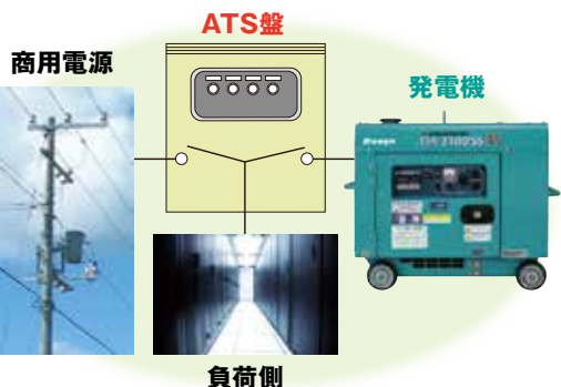
自発停型発電機※1 電源切替盤(ATS盤)※2
