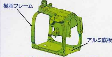
高剛性樹脂フレーム構造図
