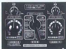
●DLW-300ESWのアークフォーストリマと1人・2人切替器
