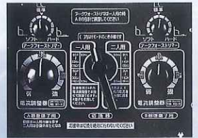
●DLW-300ESWのアークフォーストリマと1人2人切替器
